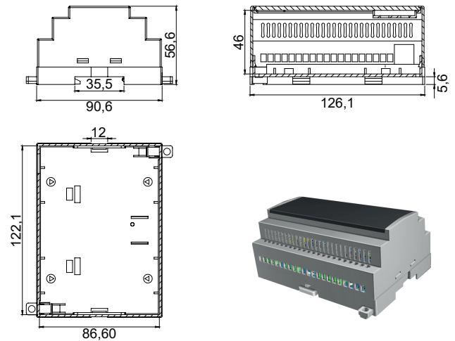
CTS 711 Montaj Şeması
