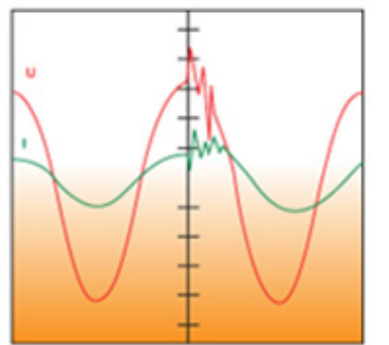
Elektromekanik Kontaktör ile Anahtarlama
